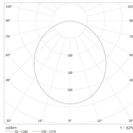
KANLUX S.A. (kat 39020) DABER 8-13W CCT W 13W / Krzywa rozsyłu światła (biegunowo)
