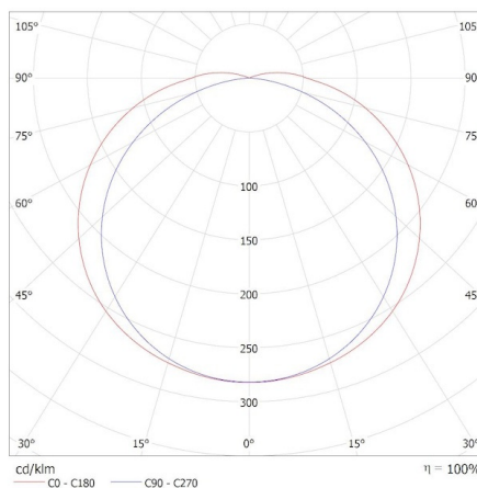
KANLUX S.A. (kat 39444) LCOB2L 28W/M24IP00-NW / Krzywa rozsyłu światła (biegunowo)
