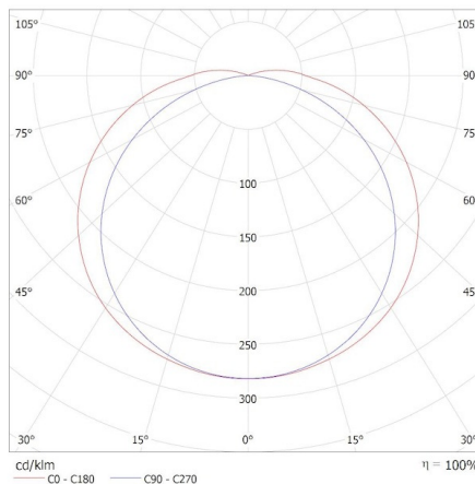
KANLUX S.A. (kat 39445) LCOB2L 28W/M24IP00-CW / Krzywa rozsyłu światła (biegunowo)
