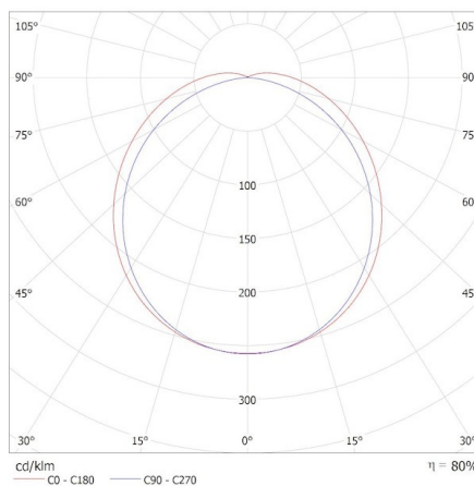
KANLUX S.A. (kat 39503) NOBEN M18W-60-CCT 15W / Krzywa rozsyłu światła (biegunowo)
