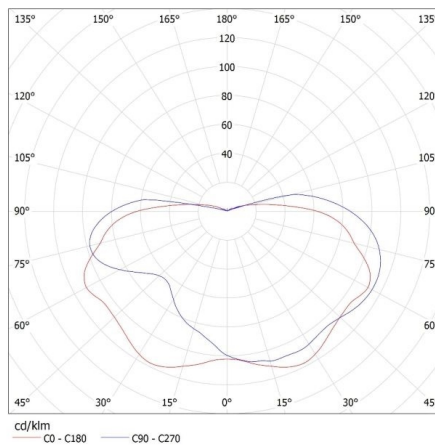
KANLUX S.A. (kat 70522) MILO 7040T / Krzywa rozsyłu światła (biegunowo)
