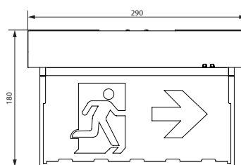
ZESTAW MONTAŻOWY ZMN
