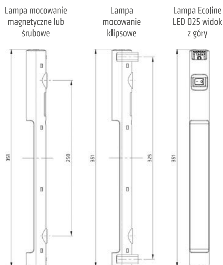
Widok boczny – montaż magnetyczny
