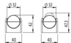
Widok boczny – montaż klipsowy
