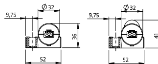
Widok boczny – montaż śrubowy
