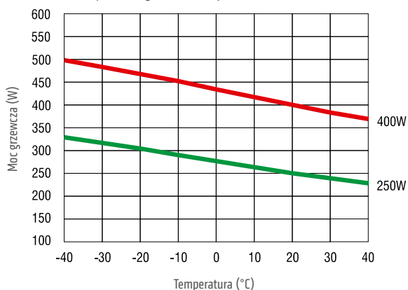
Wykres moc grzewcza / temperatura otoczenia CSF 028
