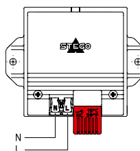
Przykład podłączenia Dmuchawa grzewcza CSF 028
