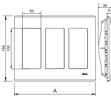
Ramka
