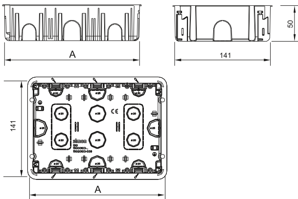
Podstawa podtynkowa
