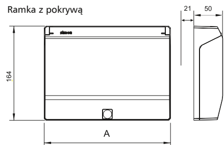
Ramka z pokrywą
