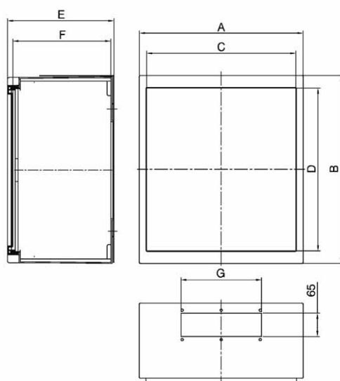
Zewnętrzne i wewnętrzne wymiary, wariant LT
