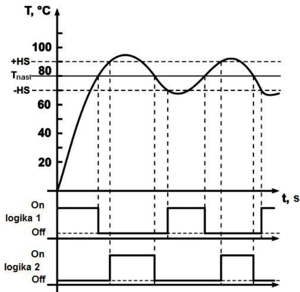
Rysunek 3.7 - Wykres zadziałania przełączników wyjściowych w trybie regulacji dwupołożeniowej
