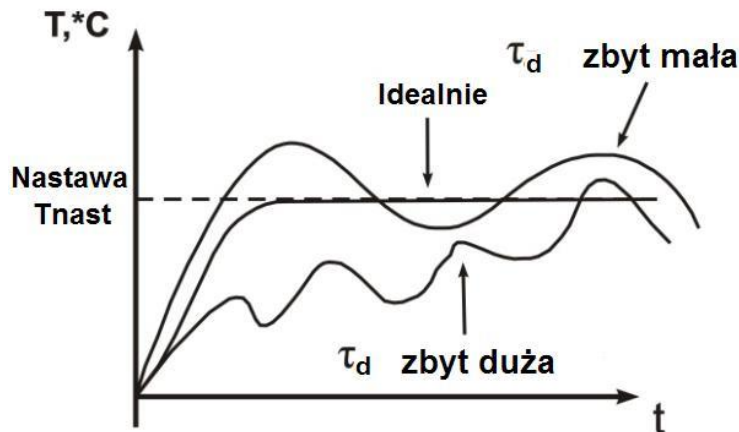
Rysunek 3.10. Wykres pracy regulatora różniczkującego
